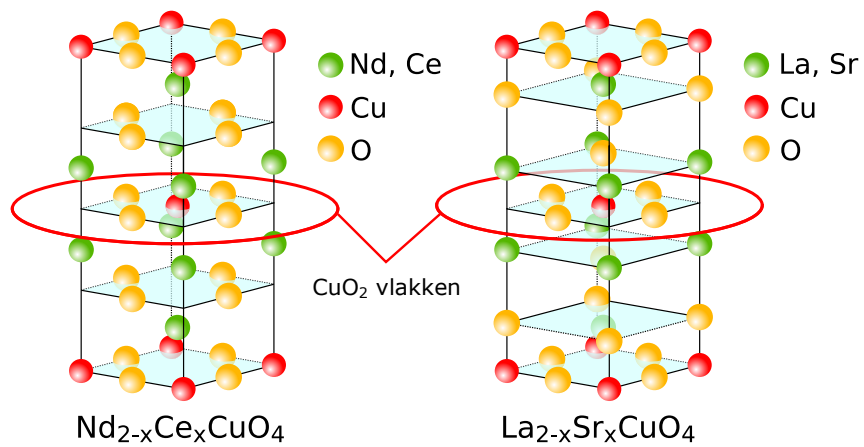
Figuur 2: De kristalstructuur van neodymiumceriumkuperoxide en lanthaanstrontiumkuperoxide, twee voorbeelden van cupraten. Ter indicatie is in beide materialen een koperoxidevlak omcirkeld. De natuurkundige eigenschappen komen voort uit de elektronen in deze koperoxidevlakken.
