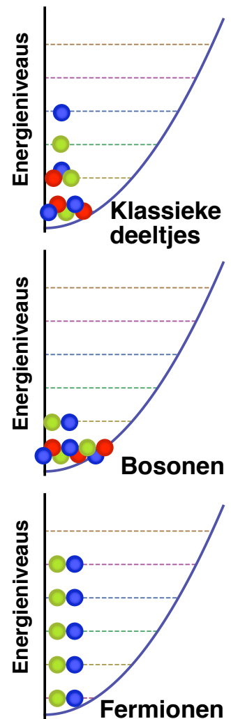
Figuur 1: Het verschil tussen klassieke deeltjes, de conformistische bosonen en de individualistische fermionen. De kleuren geven de spin van de deeltjes weer, zie voetnoot 42.
