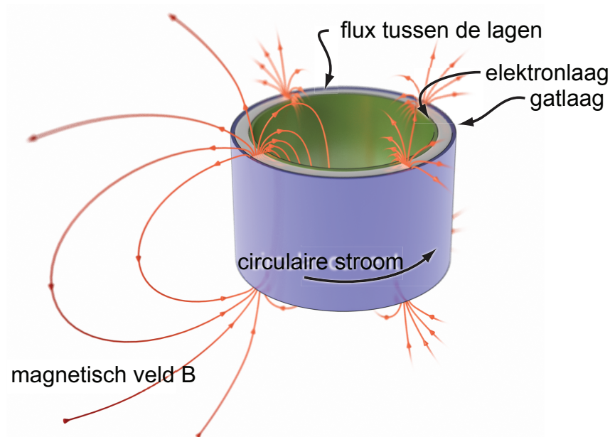
Figuur 6: Het magnetisch veld tussen de twee lagen van het dubbellaags-excitoncondensaat is gekwantiseerd.
